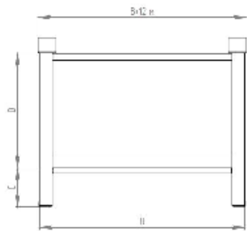
Сборочный чертеж контейнера металлического тип КГ.
