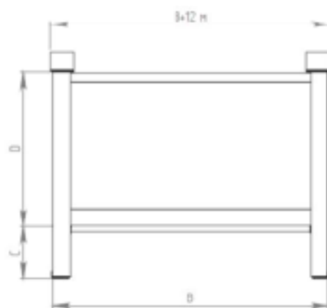
Сборочный чертеж контейнера металлического тип КГ.
