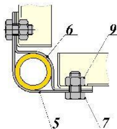
Рис. 2 Узел А
