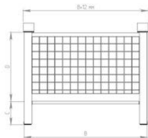
Сборочный чертеж контейнера металлического тип КС.
