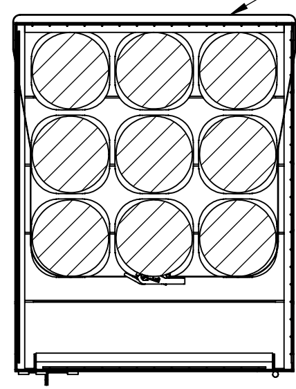
Сечение А-А Стяжной ремень
