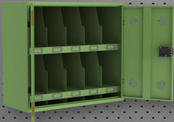
Антресошь для 10 противоголозов Арт. 036018 Габариты: 780x900x400 Размеры ячейки: 300x170x350 Вес: 41 кг
