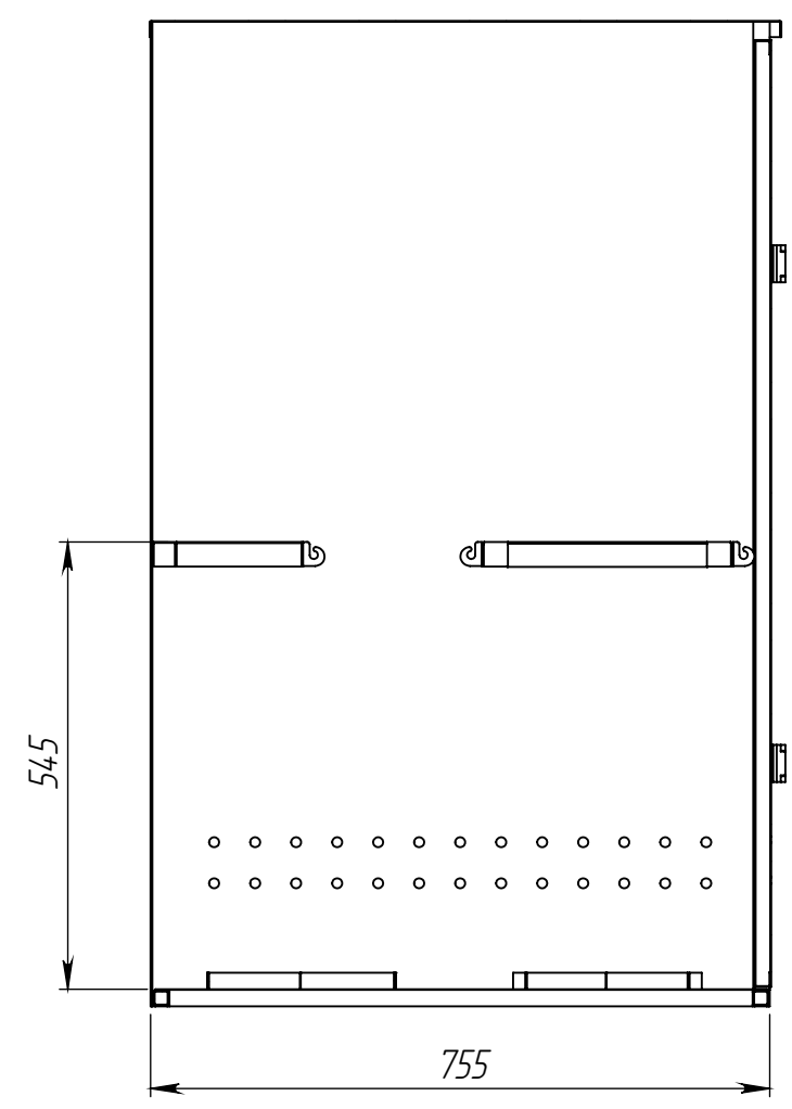
СЕЧЕНИЕ Б-Б
