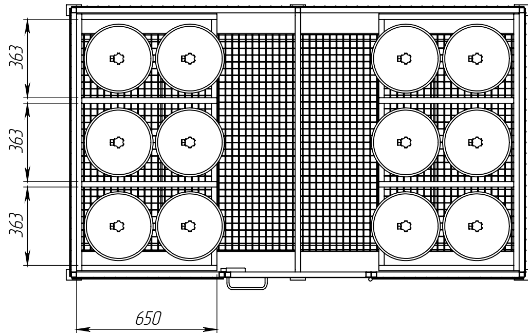
СЕЧЕНИЕ А-А
