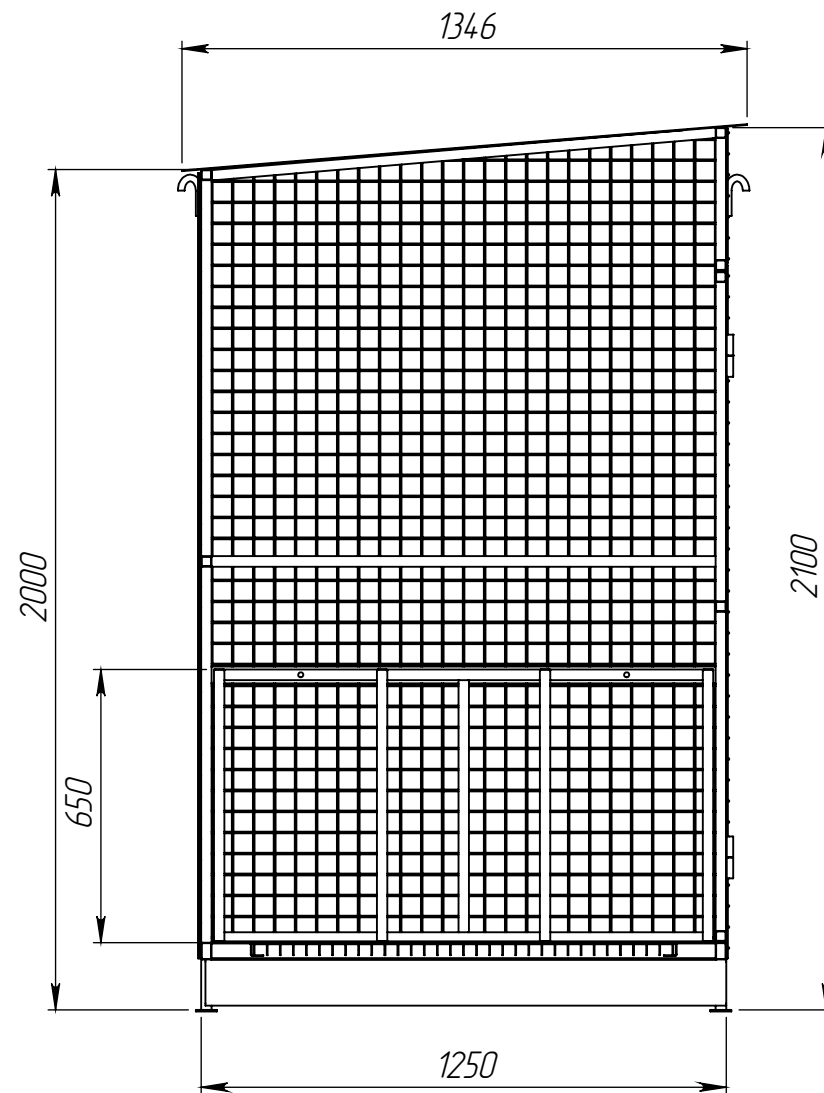
СЕЧЕНИЕ Б-Б
